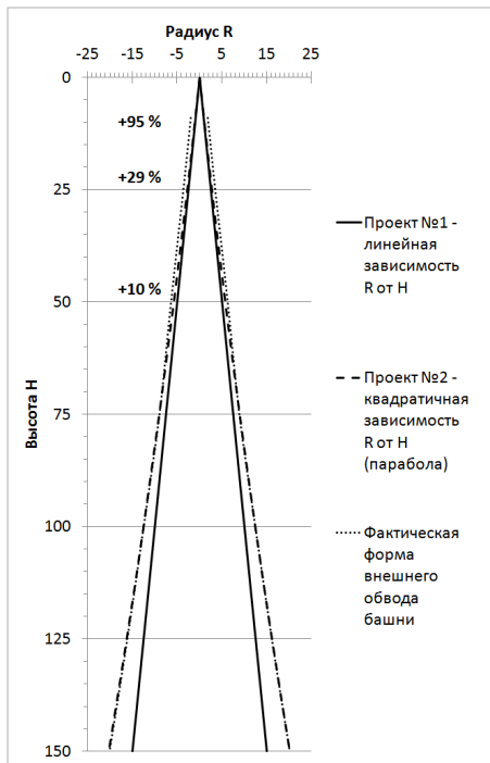
Рис. 8. Внешний обвод башни: по проектам и фактический
