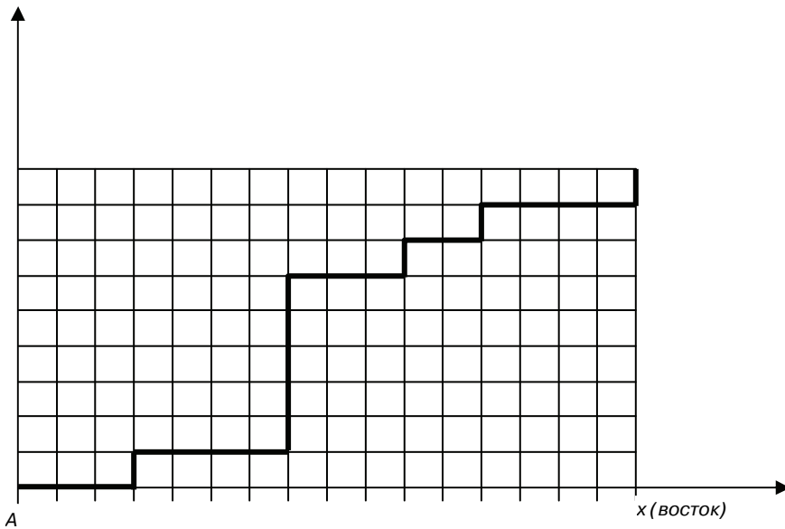
Рис. 1. Задача динамического программирования
