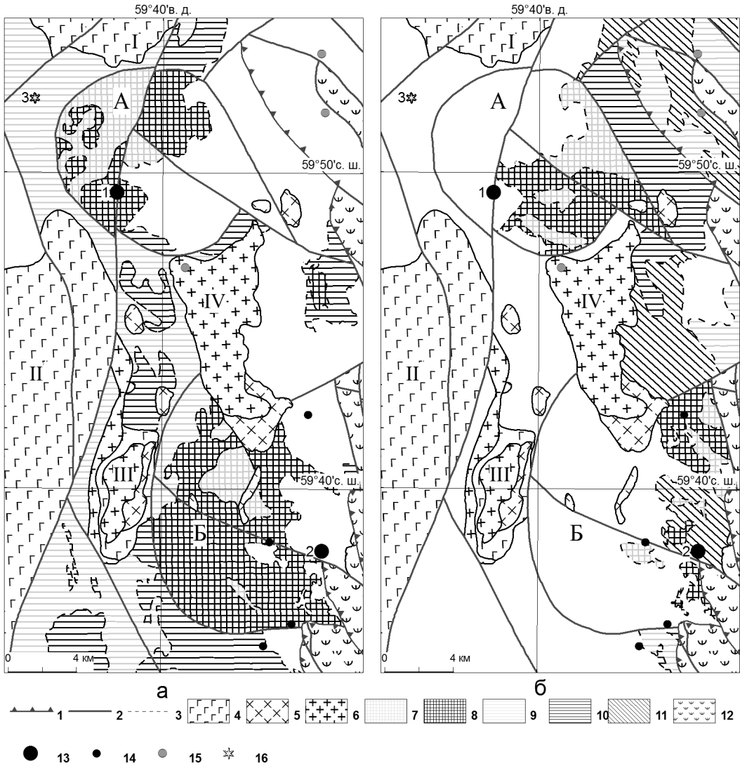
Рис. 2. Палеофациальные схемы в пределах Валенторского рудного района для шемурского (а) и павдинского (б) этапов вулканизма (с использованием данных картирования 1 : 50 000 Ю.С. Каретина и 1 : 200 000 Г.В. Петрова):
