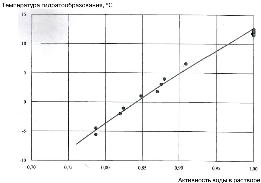
Рис. 3. Зависимость температуры гидратообразования метана от активности воды в растворе электролитов: линия — расчетные данные при давлении 9,2 МПа по доработанной методике ООО «Газпром ВНИИГАЗ»; точки — экспериментальные значения при давлениях 8,5—9,5 МПа
