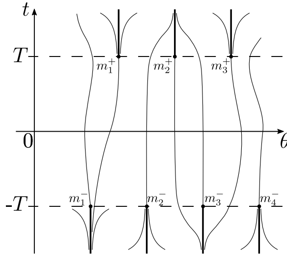
Рис. 3. Правильные переходы ИК в переходном ДУ FIG. 3. Proper transitions of integral curves in a transitional differential equation
