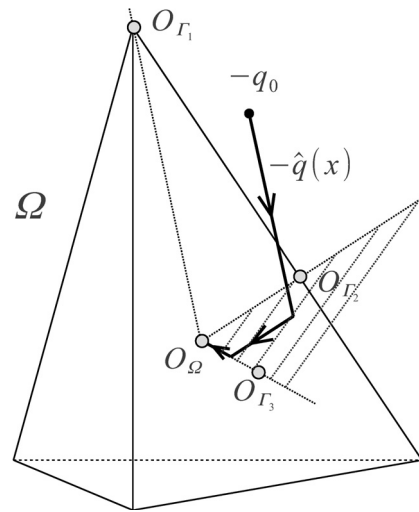
Рис. 27. Оптимальная траектория -\hat{q}(x)
